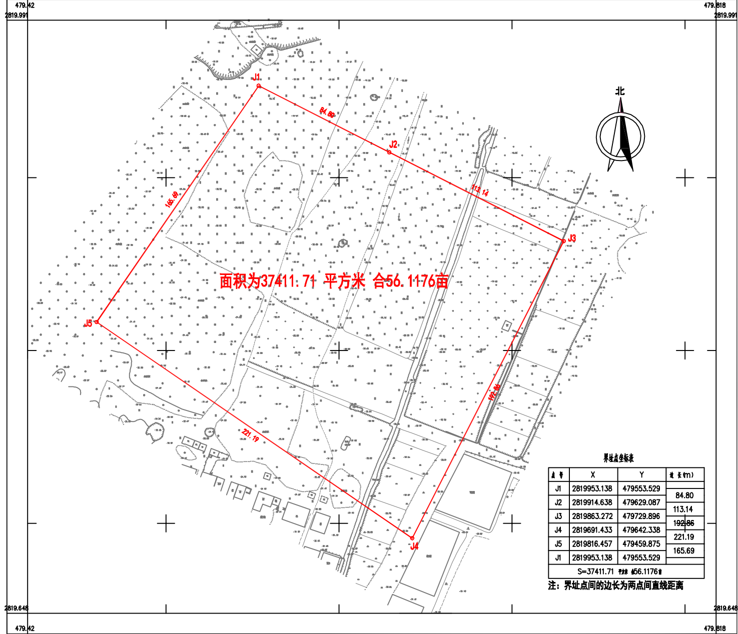
平潭龙山小学新校区选址红线图
